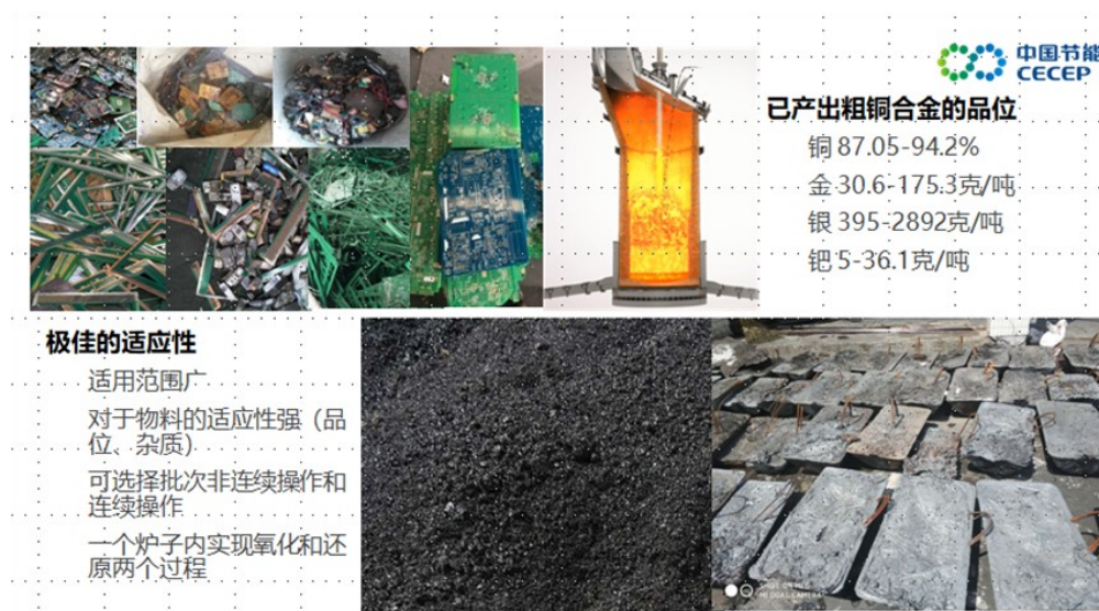
图8.2 工艺过程示意图
